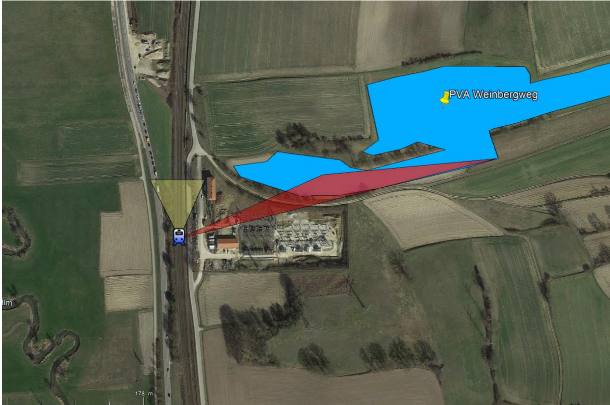
Abbildung 12: Relevanter Sichtwinkel der Zugführer auf der Bahntrasse in Gelb, Immissionswinkel möglicher Reflexionen von der Modulfläche in Rot (Quelle: Google Earth)
