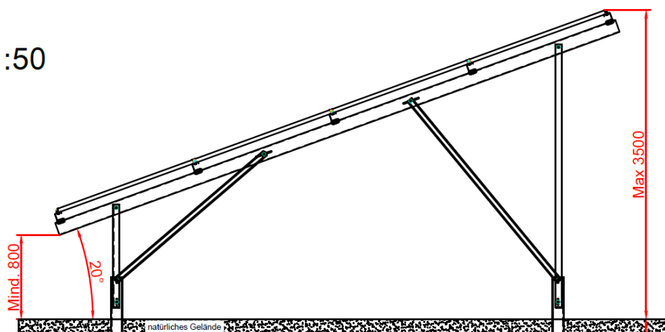
Abbildung 3: Zeichnung der Unterkonstruktion (Quelle: Auftraggeber)
