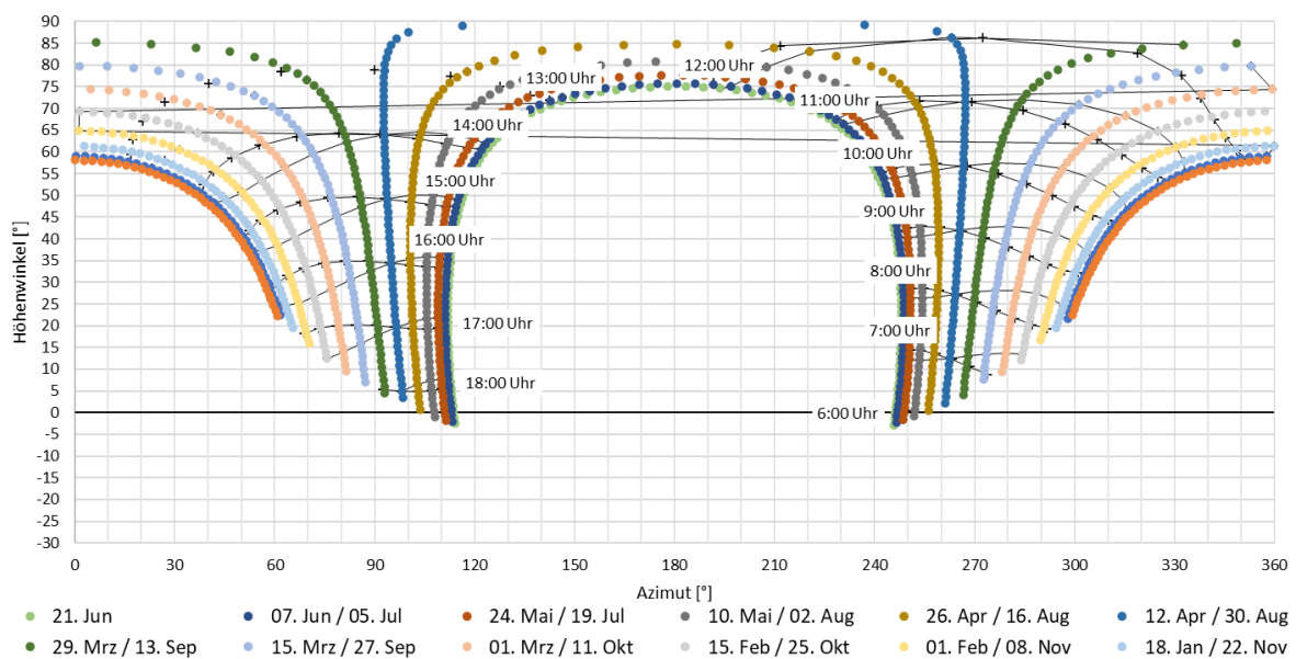
Abbildung 11: Reflexionsdiagramm der Modulfläche: 180^\circ Süd-Ausrichtung, 20^\circ Neigung, (UTC +1)
